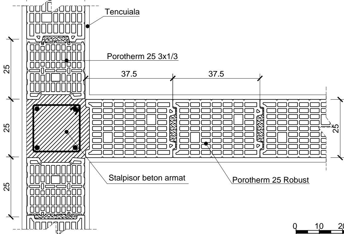
Detalii de executie zidarie confinata
